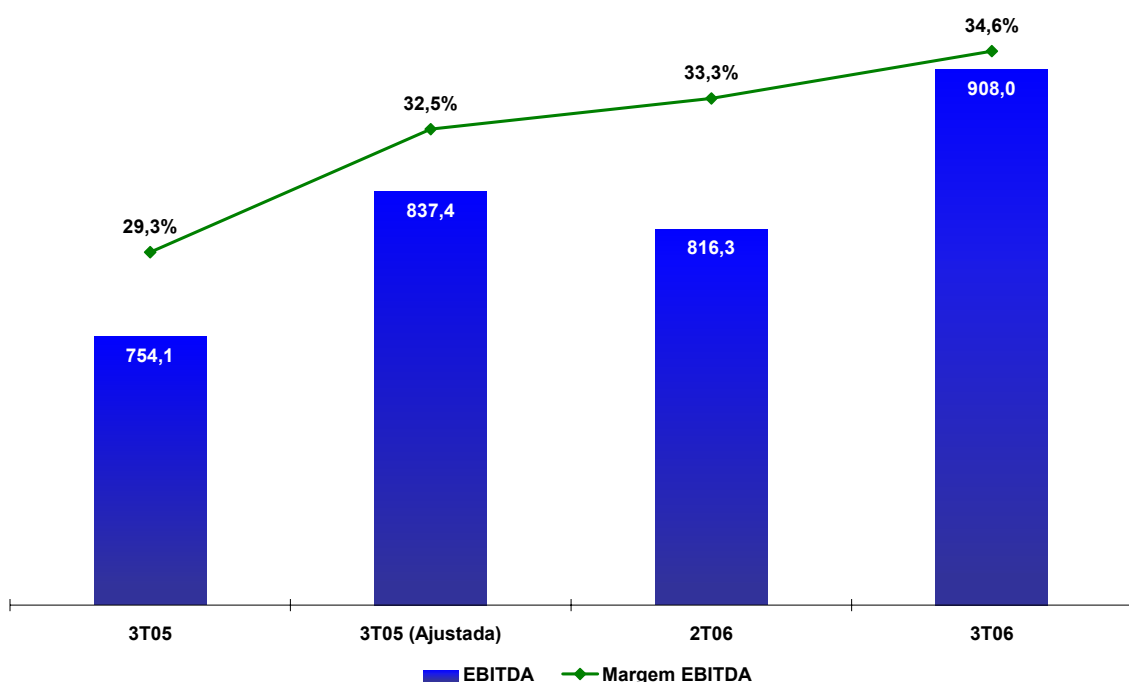
Gráfico 7 - EBITDA
